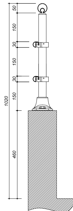
Main-courante ronde MCRØ50 2 Lisses intermédiaires MCRØ31 Fixation sur muret par sabot ELS300
